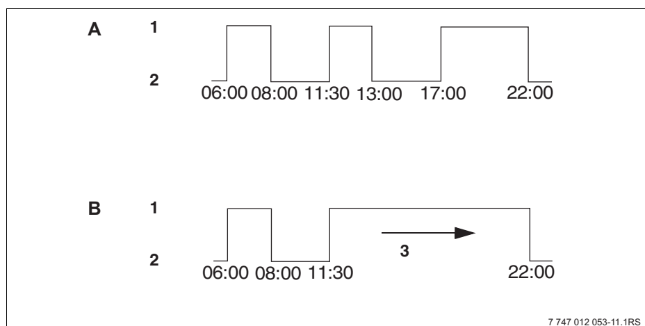
Sl. 18 Međusobno povezivanje dvije faze grijanja
