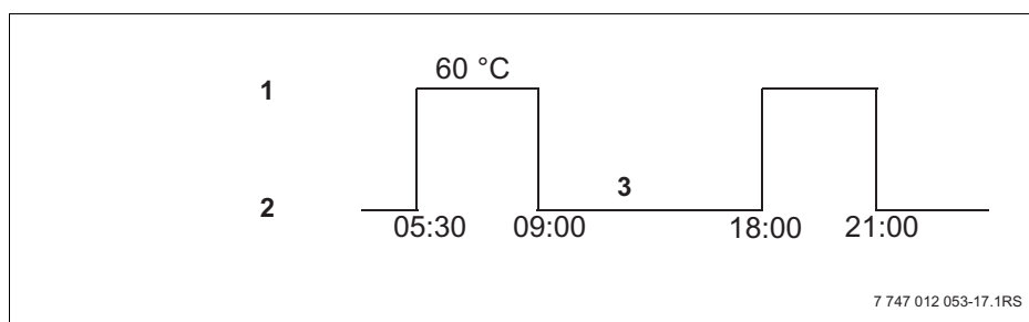
Sl. 9 Primjer: Priprema tople vode
