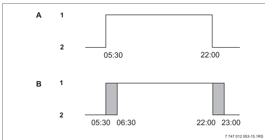
Sl. 13 Promjena uklopnih točki sa 05:30 na 06:30 i sa 22:00 na 23:00h (primjer)
