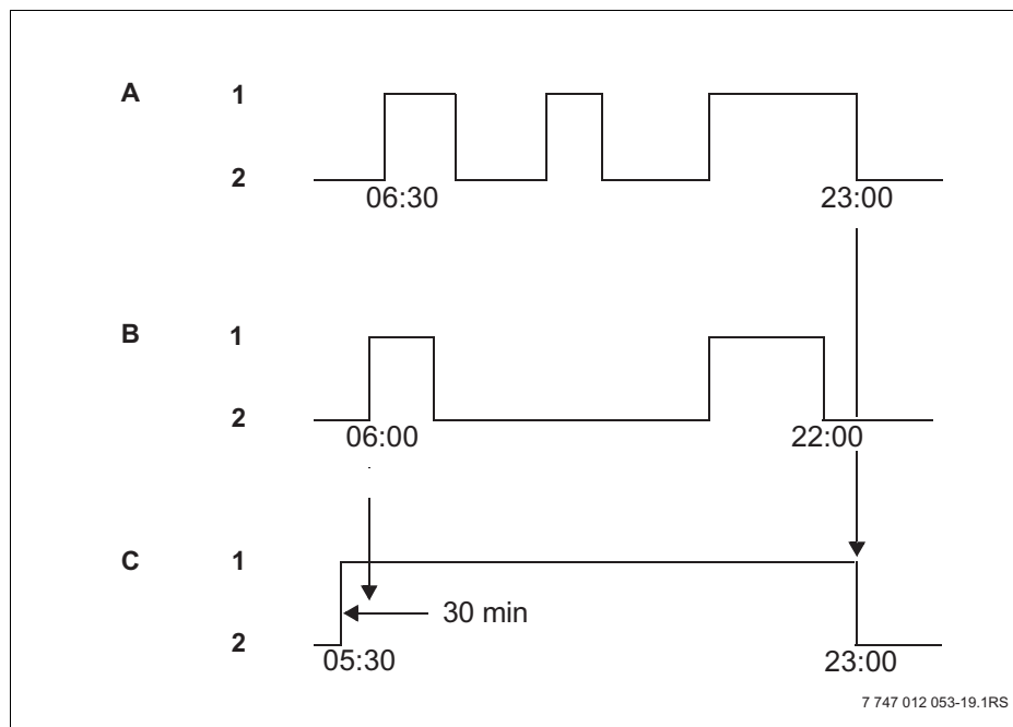
Sl. 12 Priprema tople vode počinje 30 minuta prije dnevnog pogona prvog kruga grijanja i završava s noćnim pogonom zadnjeg kruga grijanja
