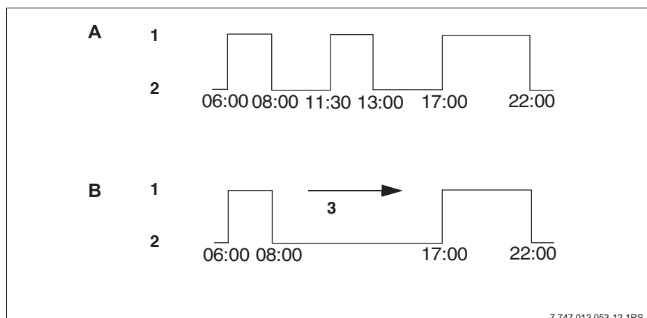
Sl. 17 Brisanje faze grijanja
