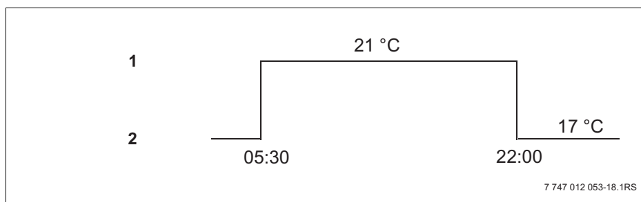
Sl. 8 Promjena sa dnevnog i noćnog pogona u fiksno utvrđena vremena na satu (primjer)
