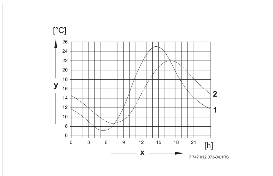
Sl. 14 Usporedba trenutačne i prigušene vanjske temperature
