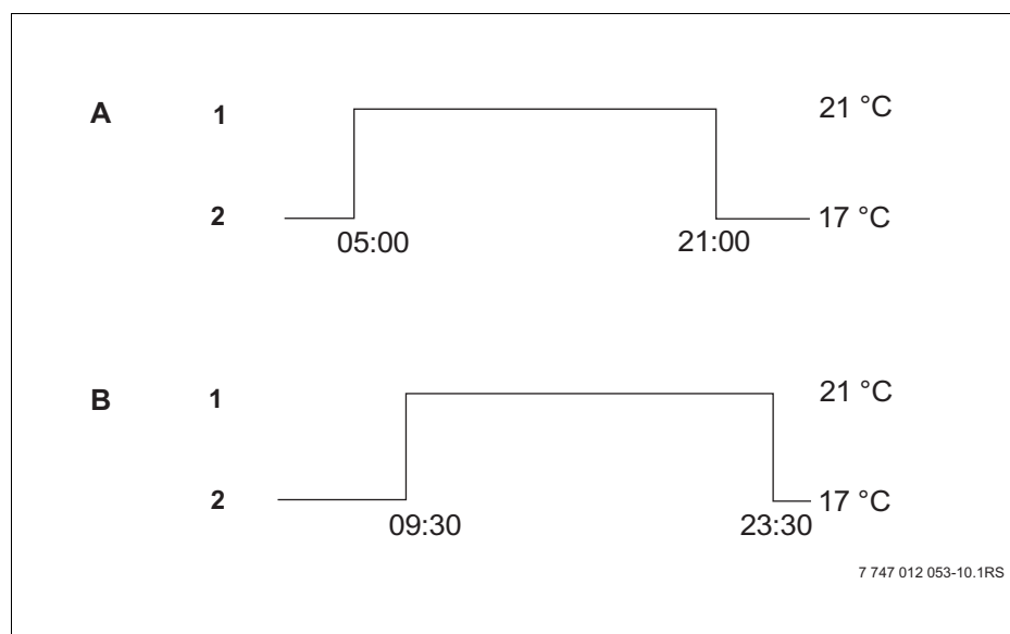
Sl. 19 Novi program grijanja
