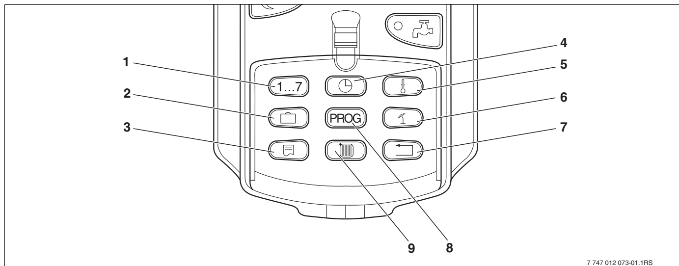
Sl. 10 Tipke za proširene funkcije
